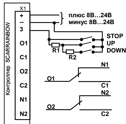
Рисунок 2. Назначение клемм электронного блока контроллера
